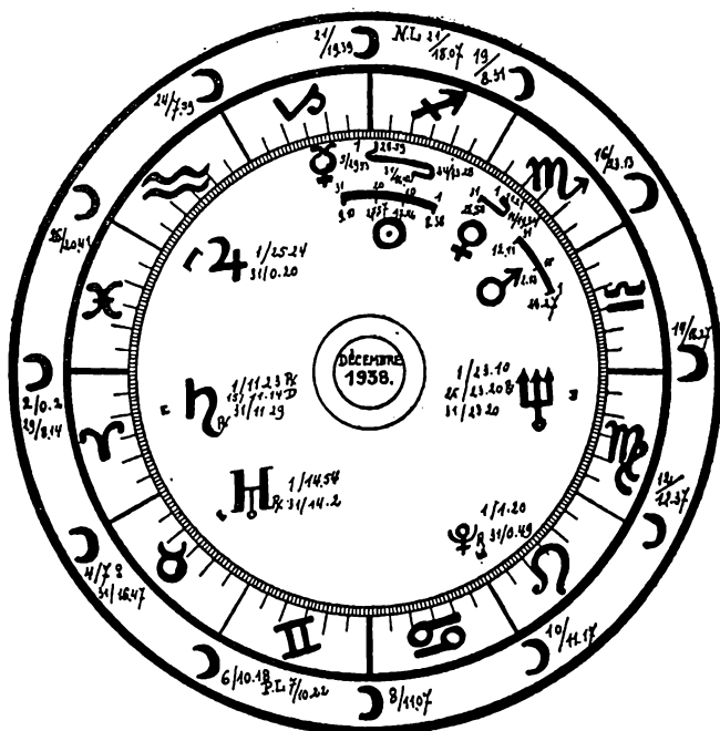
Le ciel en décembre.
